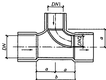
图 3 导流三通
