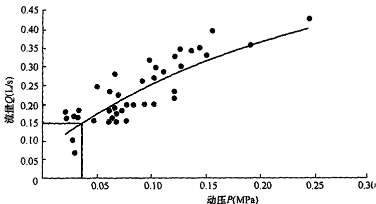
图 2 螺旋升降式水嘴半开 Q - P 曲线
