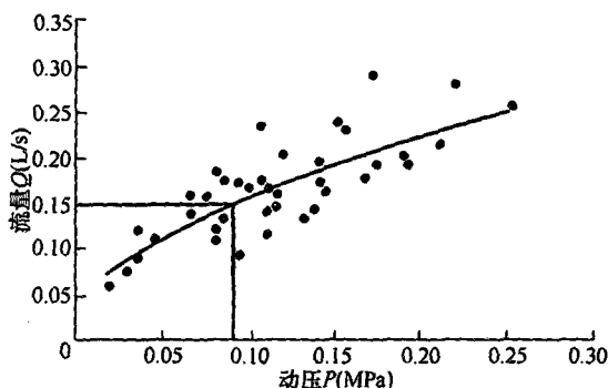
图 1 陶瓷阀芯水嘴半开 Q - P 曲线
