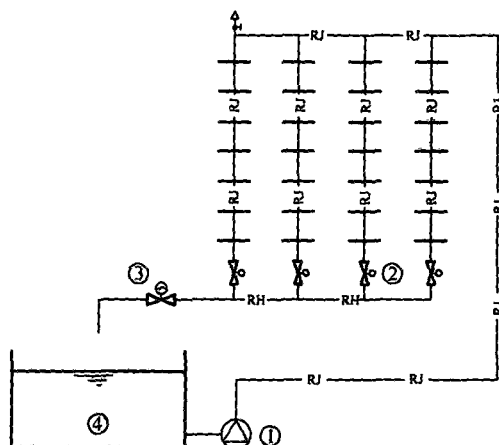
图 4 限流调节阀在热水系统中的应用
